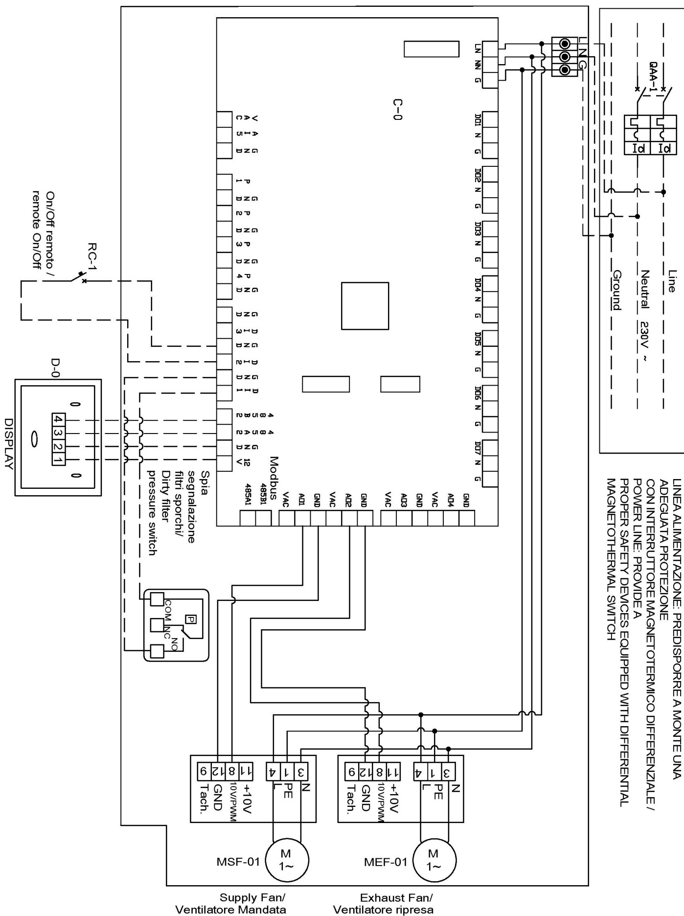
Schema elettrico CFRE+ 40N/V - 75N/V con Pannello di controllo PCUS
